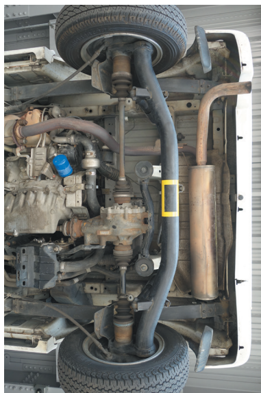
リヤ：リヤアクスルビーム
