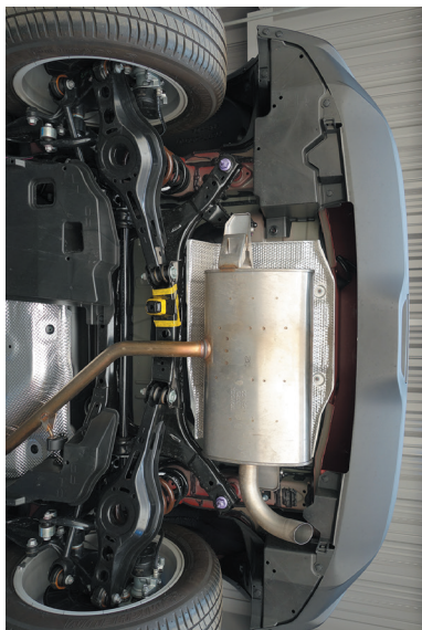
リヤ：サスペンション メンバ突起部
